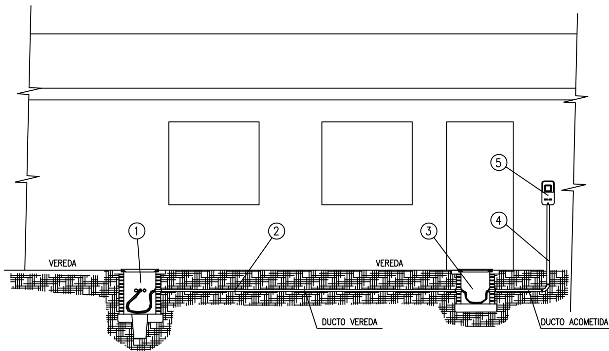
ELEVACION
